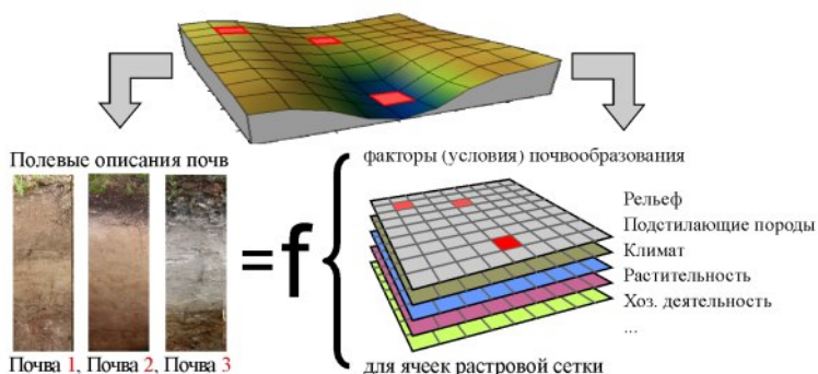
Рис. 2. Принципиальная схема цифрового почвенного картографирования на основе факторно-корреляционной модели почвенно-ландшафтных связей (Приложение 1 на цветной вкладке)
